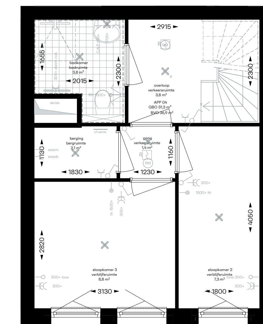
1:50 1e verdieping
