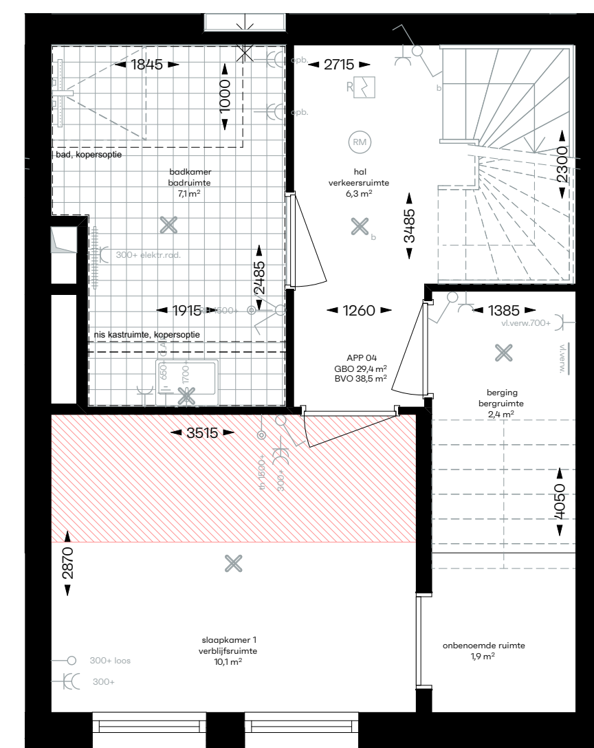
1:50 Souterrain
