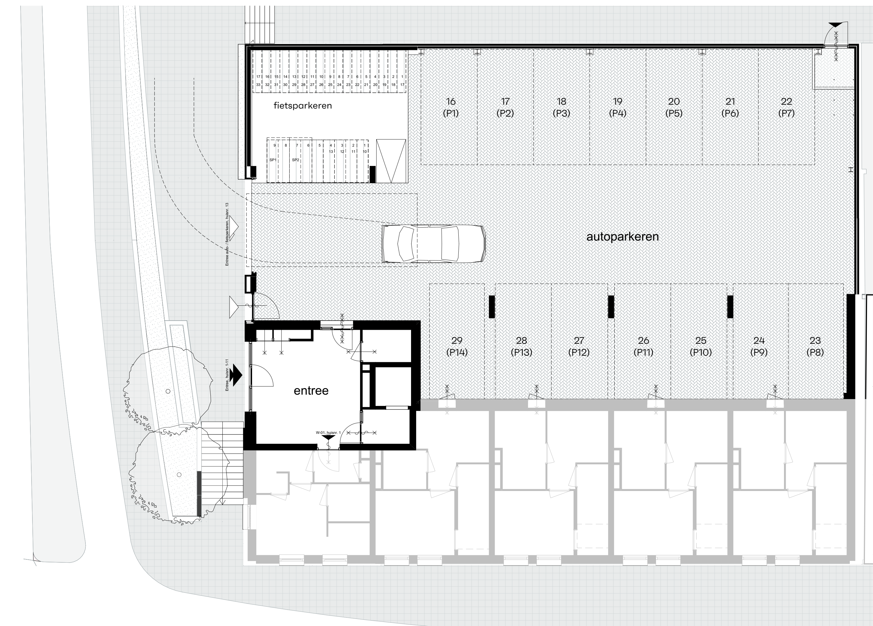
1:100 Souterrain overzicht
